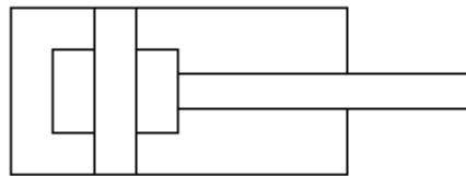
Siłownik pneumatyczny tłokowy z amortyzacją nastawną
