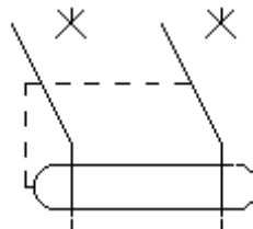
Wyłącznik silnikowy
