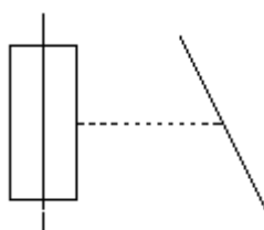
Bezpiecznik wybijakowy z oddzielnym obwodem sygnalizacji
