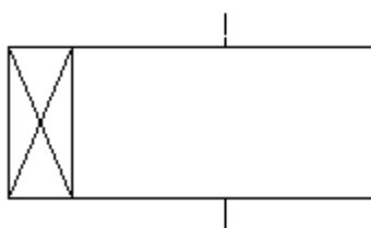
Cewka przekaźnika działającego ze zwłoką przy odwzbudzeniu i wzbudzeniu
