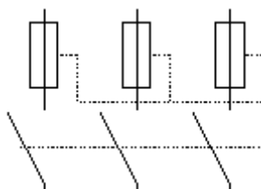
Łącznik bezpiecznikowy
