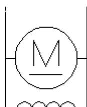
Prądnica prądu stałego szeregowo-bocznikowa
