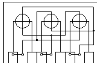
Licznik 3-fazowy podłączenie pośrednie
