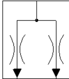
Regulator przepływu - nastawialny
