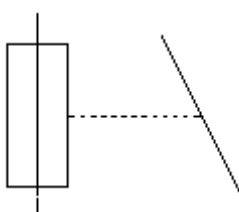
Łącznik trójfazowy z samoczynnym wyzwalaniem spowodowanym zadziałaniem któregokolwiek z bezpieczników
