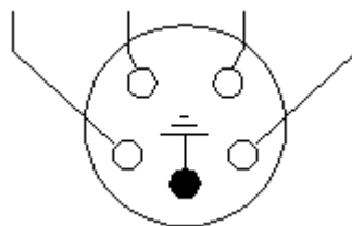
Gniazdo 3F+E
