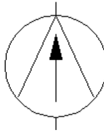
Sprężarka wyporowa
