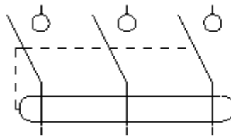
Rozłącznik bezpiecznikowy
