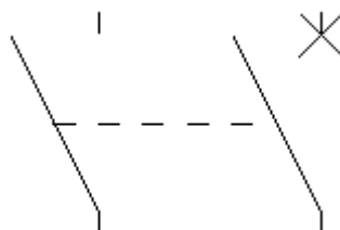
Wyłącznik 1+N
