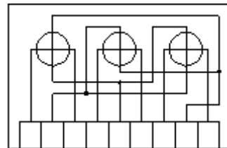
Licznik dwutaryfowy podłączenie bezpośrednie
