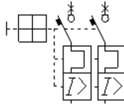
Włącznik silnikowy
