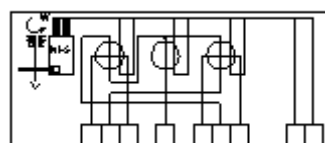
Licznik maksymalny podłączenie pośrednie
