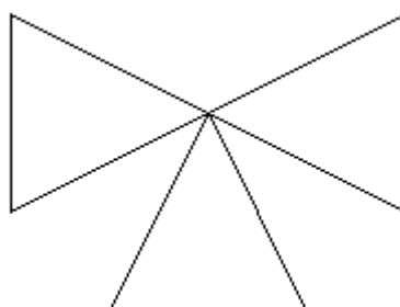
Zawór grzybkowy trójdrożny
