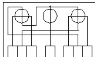
Licznik energii biernej z nadajnikiem impulsów
