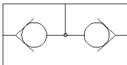
Zawór koniunkcji
