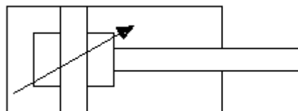
Siłownik pneumatyczny z tłokiem dwustronnym
