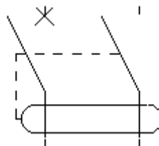
Wyłącznik różnicowy
