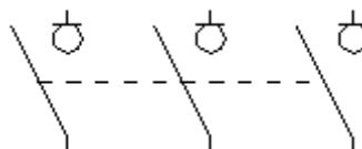
Rozłącznik izolacyjny bezpiecznikowy
