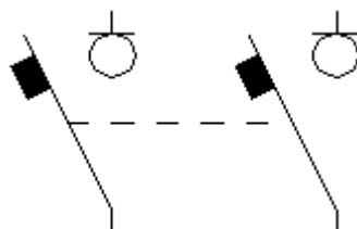
Stycznik
