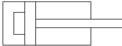
Siłownik pneumatyczny tłokowy z amortyzacją dwustronną
