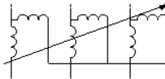
Przekładnik prądowy dwurdzeniowy
