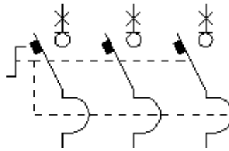
Wyłącznik silnikowy
